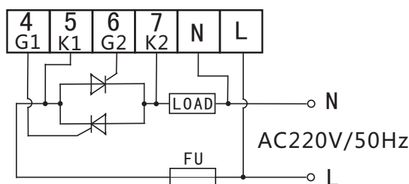
ZKD-3A调整器接线图
